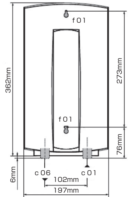
前面透視図
